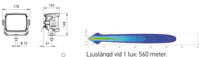
Ljuslängd vid 1 lux: 560 meter.
