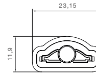
Abmessung Endkappe Dimension endcap
